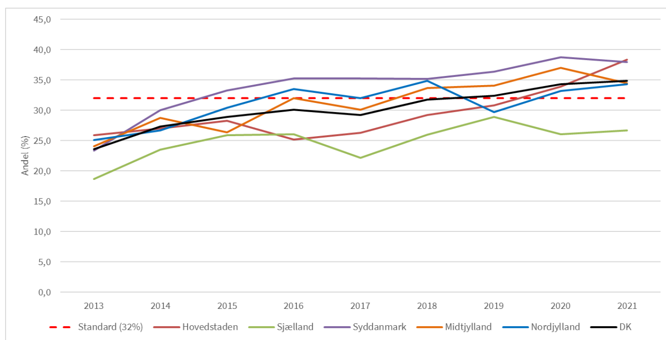
Figur 3.5.2: Trend for indikator Va efter patientens bopælsregion ved diagnose, 2013-2021
